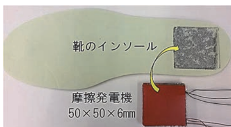
図2. インソール組込み摩擦発電機
