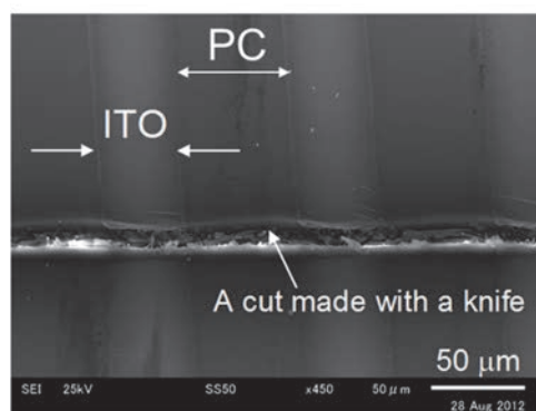
ポリカーボネートの表面にリボン状にパターンニングした導電性ITO薄膜
