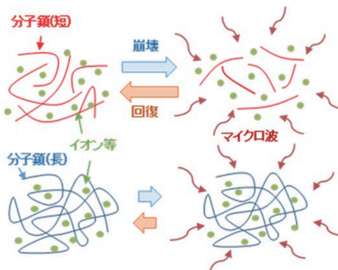
図2 マイクロ波によるクラスター崩壊イメージ
