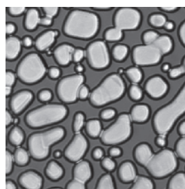
図2 冷却後の氷結晶の様子
