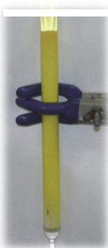
希薄水溶液からのCr(VI)の連続除去装置
