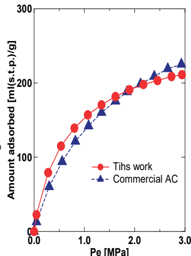
Fig. 活性炭へのメタンの吸着等温線（吸着温度25℃）
