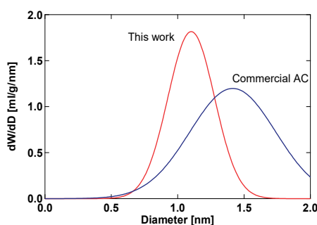
Fig. 活性炭のミクロ孔分布（市販品との比較）
