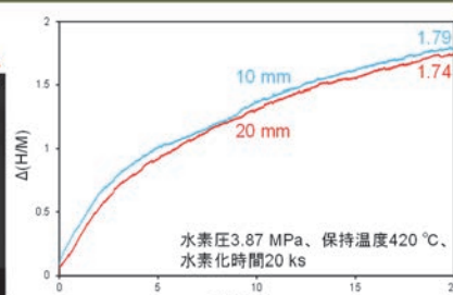
図 Φ0.5 (A) Mg/Fe複合線材 水素吸蔵量
