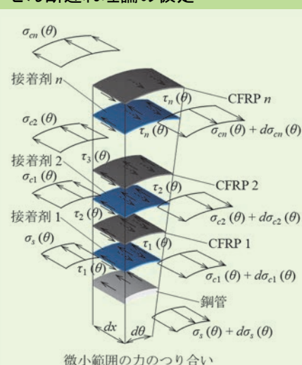
せん断遅れ理論の仮定
