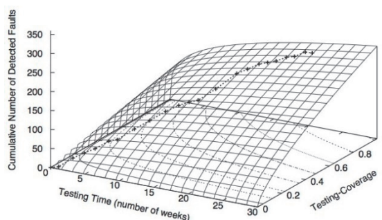
推定された2変量ワイブル型信頼度成長モデル
