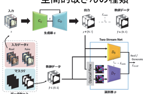
GANを用いた手法 [1]
