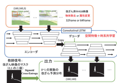
Convolutional LSTMを用いた手法 [3]
