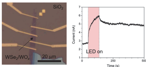
図1. 表面酸化したWSe 2 原子層を用いた光センサー
