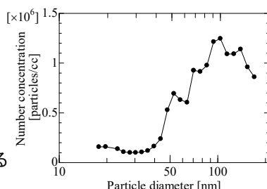
Fig. 2 衝突前の凝集粒子の粒径分布
