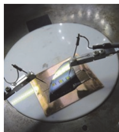
図. 電圧印加の実験装置
