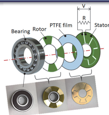
図1. 摩擦帯電センサ組み込み軸受
