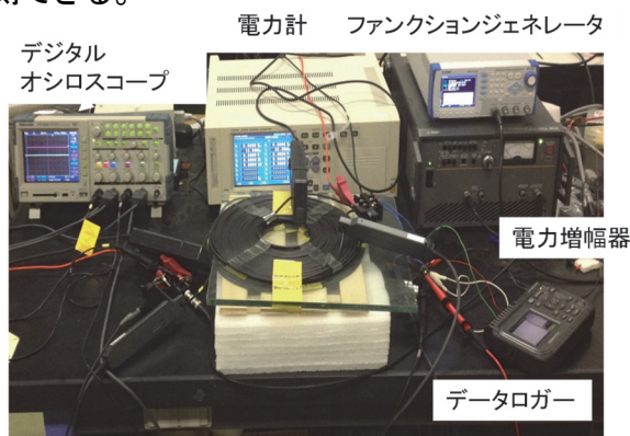
非接触充電装置の電力伝送実験装置と電力伝送効率の測定・解析結果
