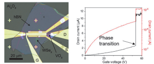
図2. 相転移材料VO 2 を電極とするWSe 2 原子層FET
