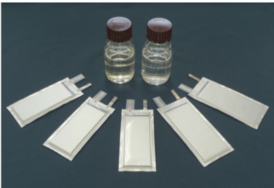
EMIFSIイオン液体(瓶中)とそれを用いた「初めての純イオン液体リチウムイオン電池」 FC EXPO 2009および2011 NEDOブース展示
