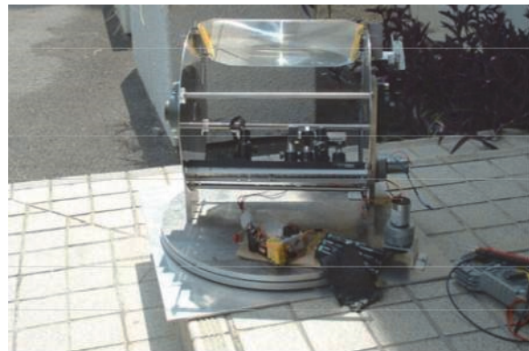
太陽光直接励起レーザー装置
