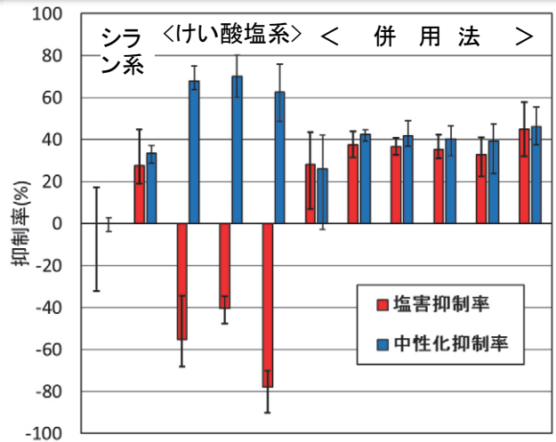
図2 塩害と中性化が生じる条件での抑制率
