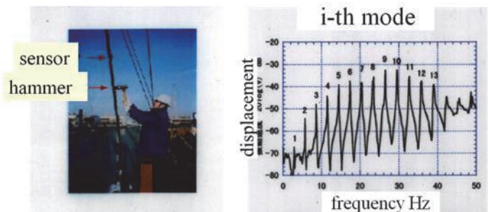
橋梁ケーブルの打撃試験と複数個の共振周波数
