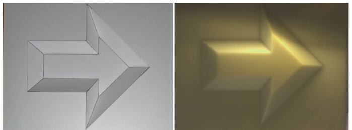
【ホロウマスク錯視の例】
