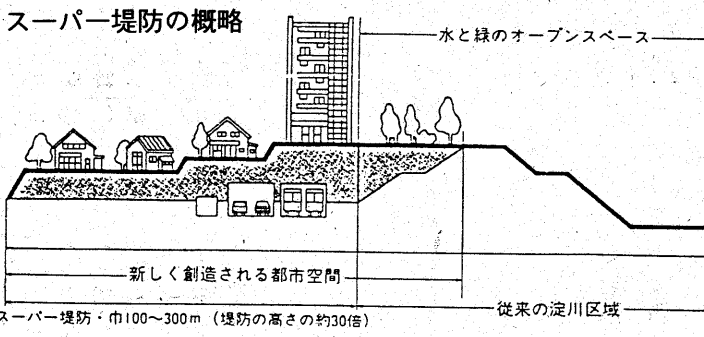
スーパー堤防の概略
