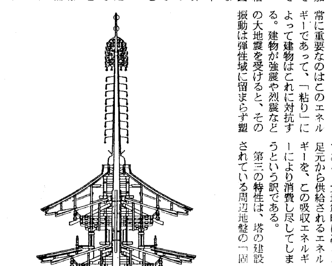
醍醐寺五重塔(工学部水防振男教授提供)
