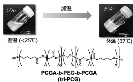
図 1. 本研究で基材として使用している生分解性インジェクタブルポリマー PCGA- b -PEG- b -PCGA (tri-PCG)。
