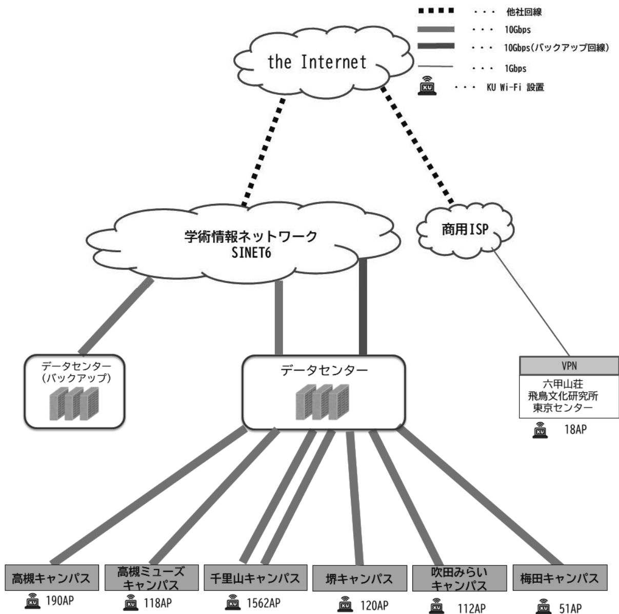
関西大学学術情報ネットワーク構成図 【KAISER】
