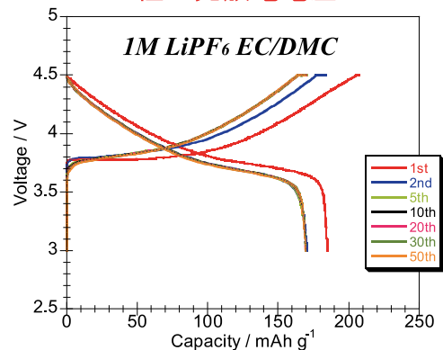
開発 水系バインダーで作成した NMC正極の充放電電圧カーブ
