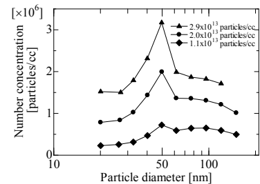
Fig. 3 分散化した50nmの非凝集粒子ピークを示す衝突後の凝集粒子粒径分布
