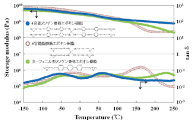
図1. 4官能性メソゲン骨格エポキシ樹脂の動的粘弾性
