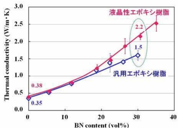
図1 BNフィラー充填に伴うコンポジットの熱伝導率変化
