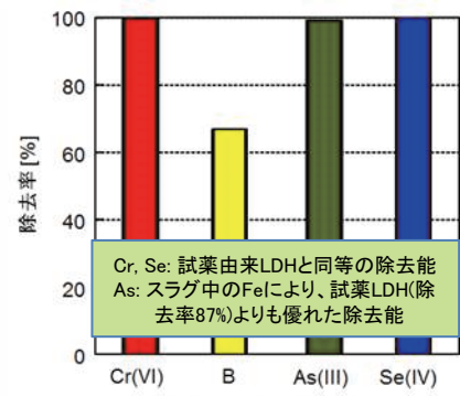
図2 スラグ由来LDHによる陰イオン種の除去 出発原料: 製鋼スラグ, 初期濃度: 20ppm Cr, Se: 試薬由来LDHと同等の除去能 As: スラグ中のFeにより、試薬LDH(除去率87%)よりも優れた除去能
