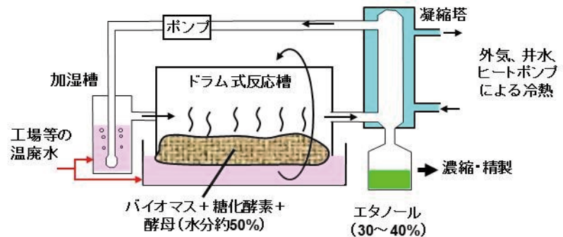
ドラム式反応槽(容量50L)
